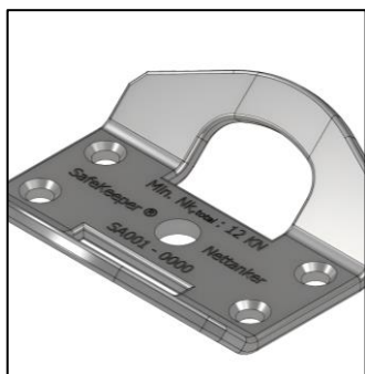
Nettanker SA001 Festekrok til montering av nett
