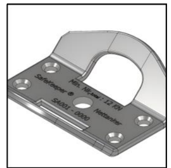
Nettanker SA001 Festepunkt til montering av nett
