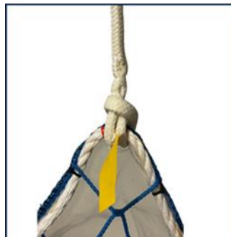
SN9001/9002 Opphengslinje 3/13,5 m 12mm tau med øye
