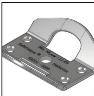
SA001 Nettanker Opphengspunkt for montering av nett
