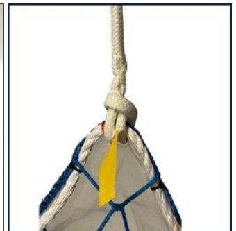
Opphengsline 3 / 13,5 m SN9001 / 9002 12 mm tau med øye, 30 kN
