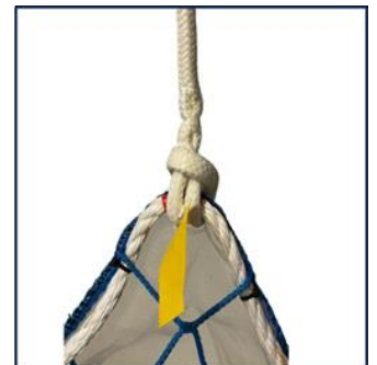
Opphengslinje 3/13,5 m SN 9001/9002 12 mm tau med øye, 30 kN
